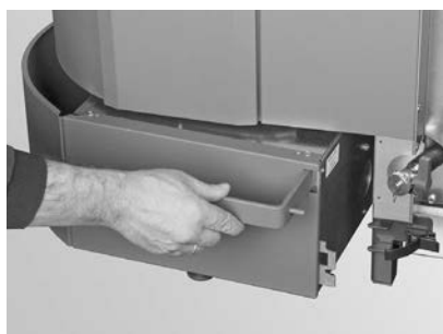
rys.32 Pchnij popielnik lekko w lewo
