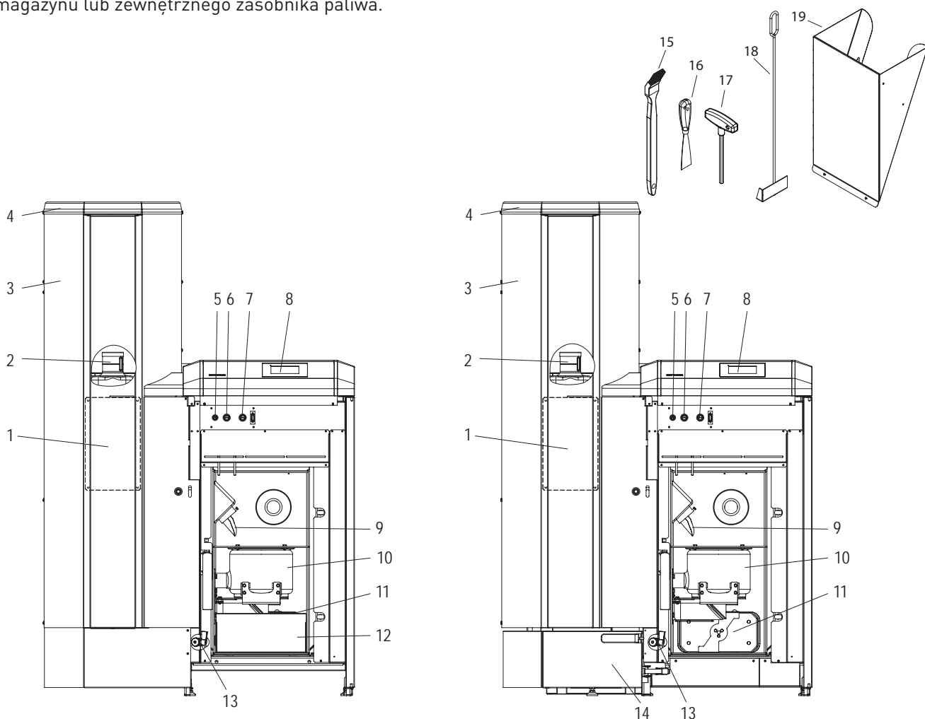
rys. 12 BioWIN 2 Touch Premium bez drzwiczek zewnętrznych oraz drzwi komory spalania
