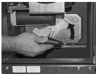
rys. 29 Przekręć uchwyt w stronę przeciwną do ruchu wskazówek zegara
